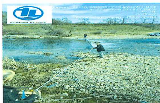
Gypi i dëmtuar i Çelikut Ø 300, në Lumin Ibër, fshati Vinarc.
