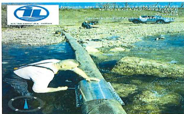
Gypi i dëmtuar i Çelikut Ø 300, në Lumin Ibër, fshati Vinarc.
